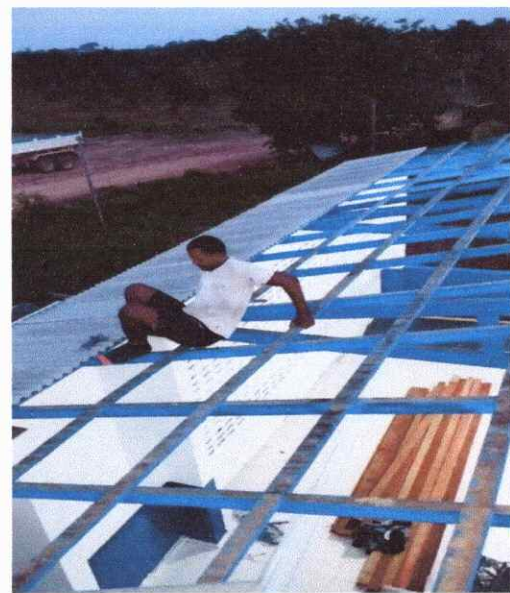
FOTO 138 EXECUÇÃO DE TRAMA E TELHAMENTO
