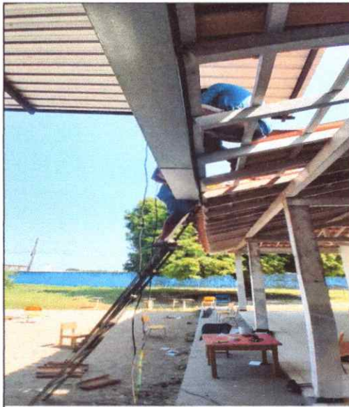
FOTO 35 INSTALAÇÃO DE CALHA EM CHAPA DE ZINCO
