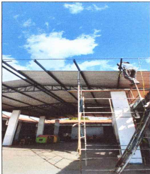
FOTO 13 MONTAGEM ESTRUTURA COBERTURA
