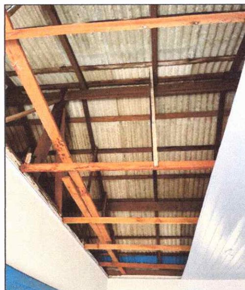
FOTO 94 ANTES DA MANUTENÇÕES
