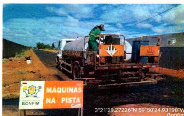
PAVIMENTAÇÃO Pintura de Ligação
